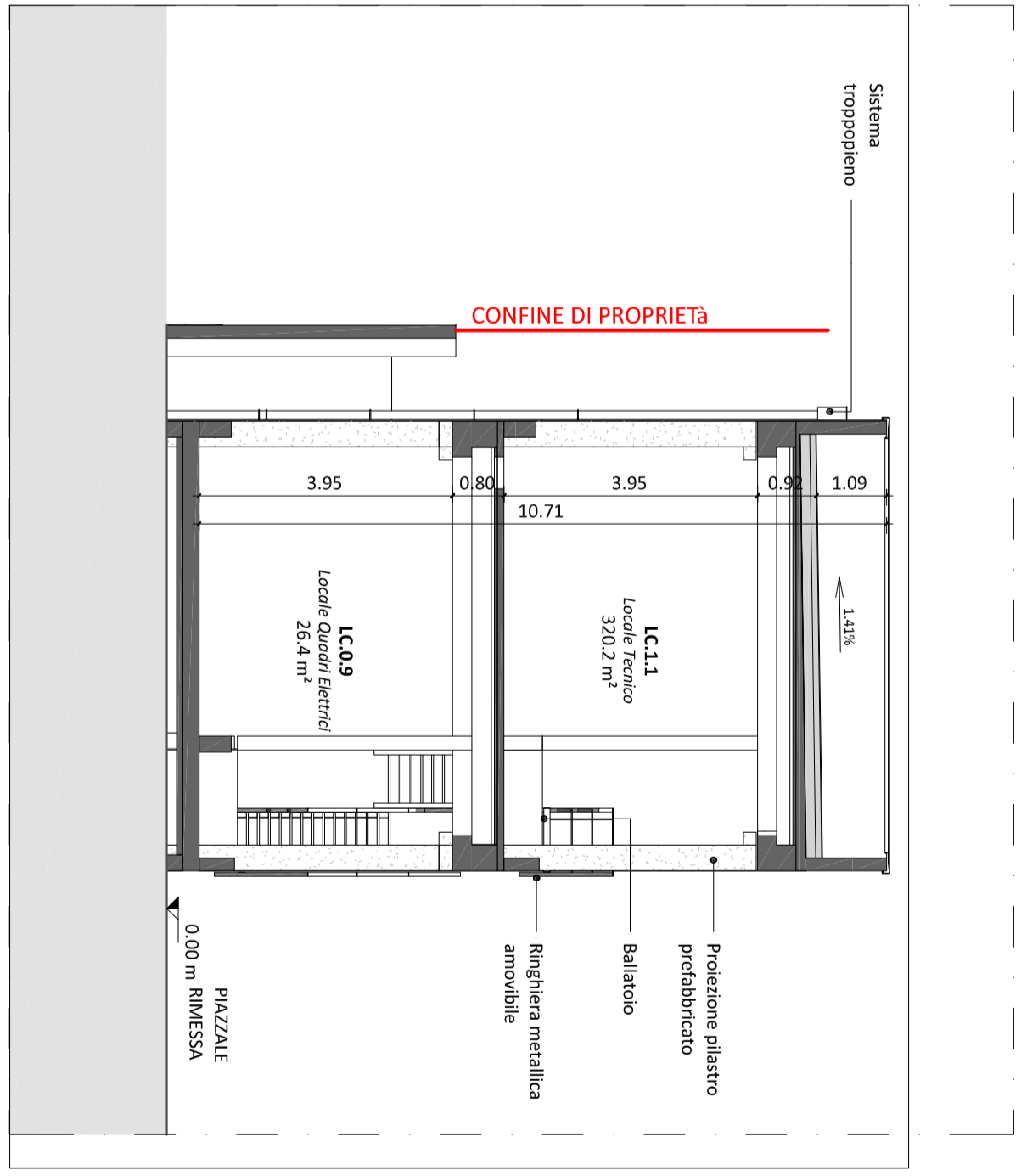
Locale Charger - Sezione F 1:100
